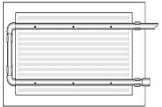
标准的回风口采样
